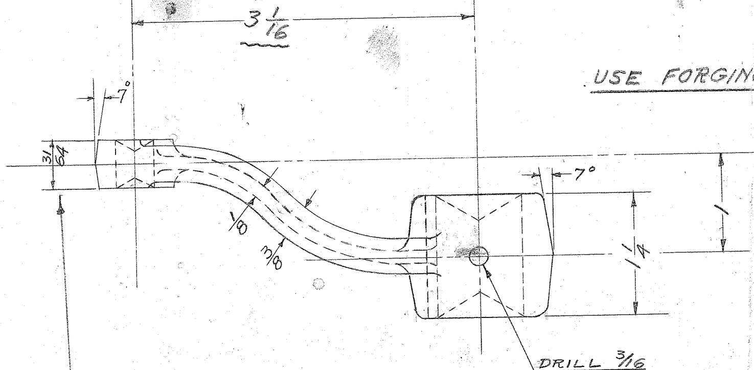
SECTION A-B
